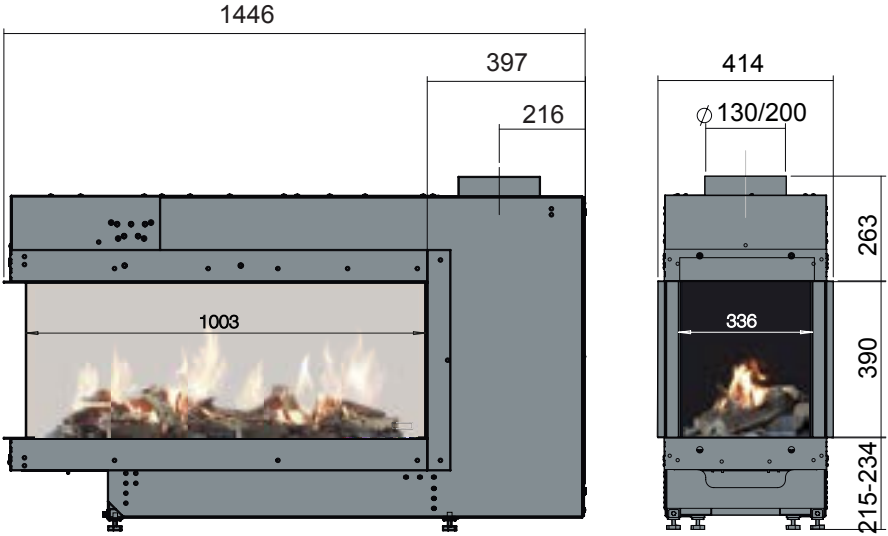
Chimenea a Gas|FABER (NL)| ASPECT PREMIUM RD L
